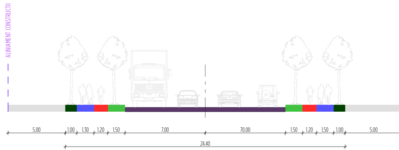
PROFIL TRANSVERSAL - STRADA CATEGORIA II
