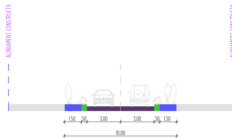
PROFIL TRANSVERSAL - STRADA CATEGORIA IV (DRUMURI INTERIOARE ZONA I1a)
