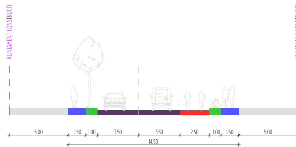
PROFIL TRANSVERSAL - STRADA CATEGORIA III
