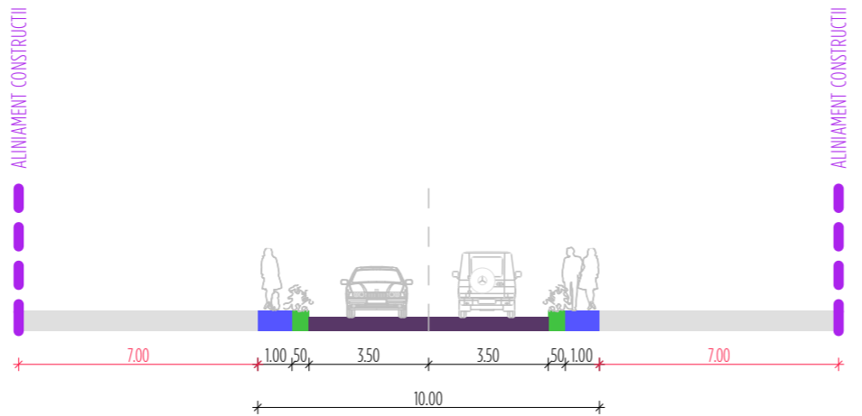
PROFIL TRANSVERSAL - STRADA CATEGORIA IV (DRUMURI INTERIOARE ZONA L1a)
