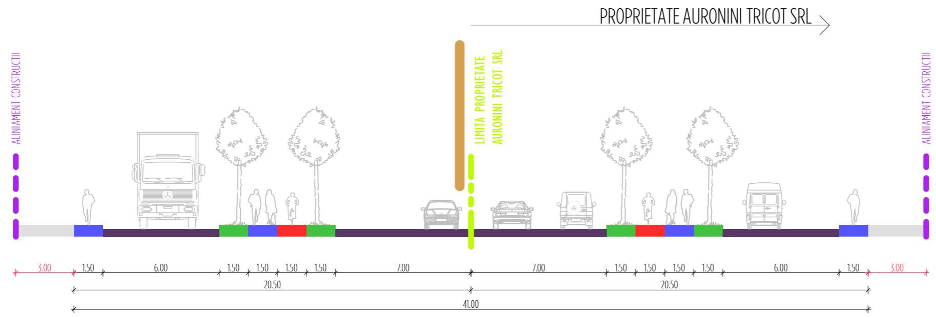
PROFIL TRANSVERSAL - "ORBITAL" - EXTINDERE SOSEAU DE CENTURA - STRADA CATEGORIA II
