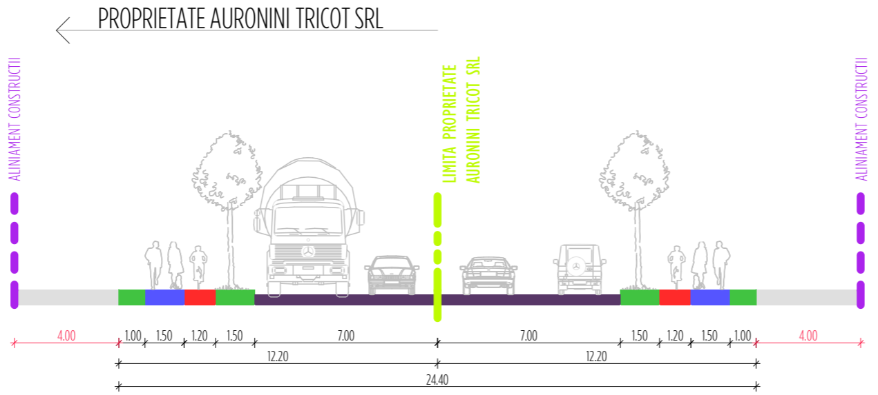
PROFIL TRANSVERSAL - STRADA CATEGORIA II
