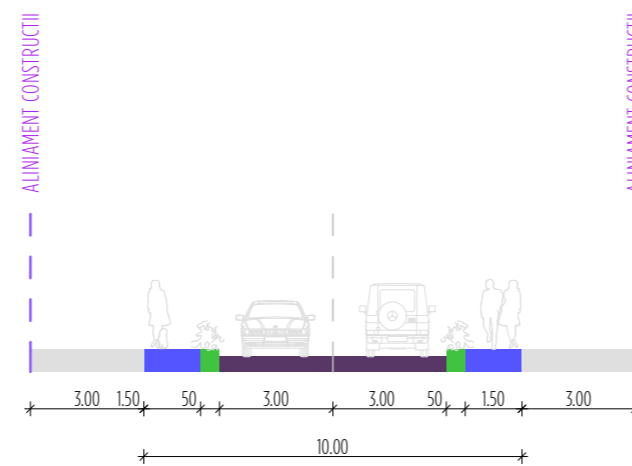
PROFIL TRANSVERSAL - STRADA CATEGORIA IV
