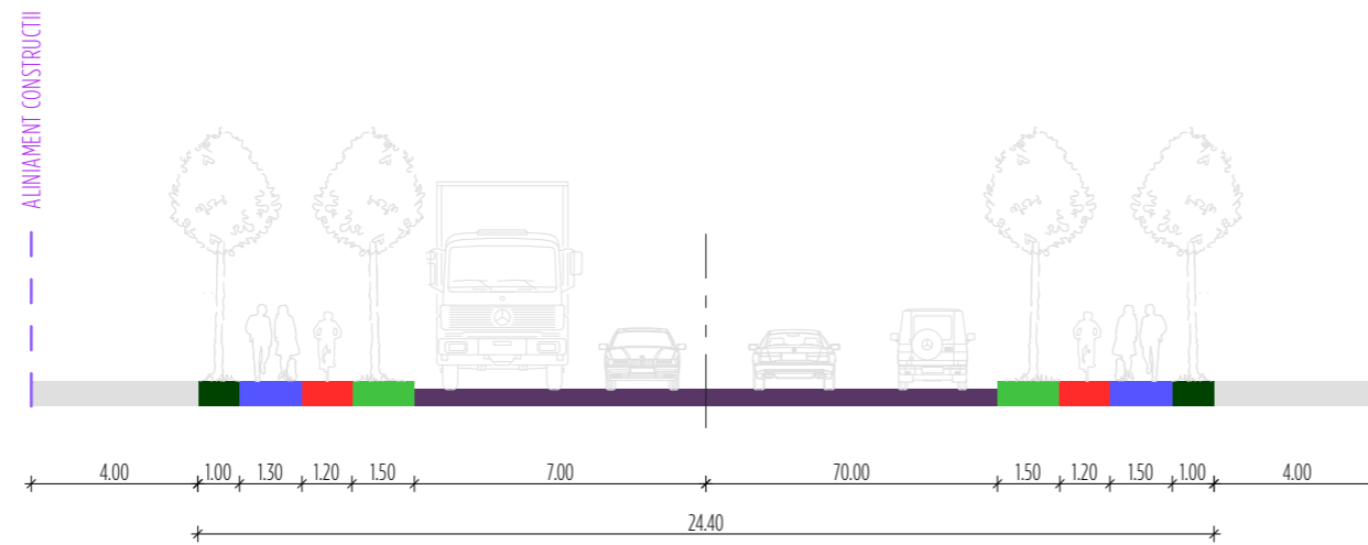
PROFIL TRANSVERSAL - STRADA CATEGORIA II
