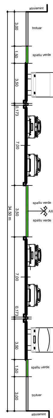
SECTIUNEA A - A PROFIL TRANSVERSAL STRADA CAT. II
