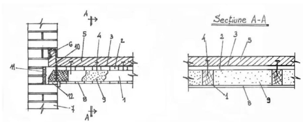
Detaliu 2 - introducerea planseului din beton armat peste planseul din lemn existent.
