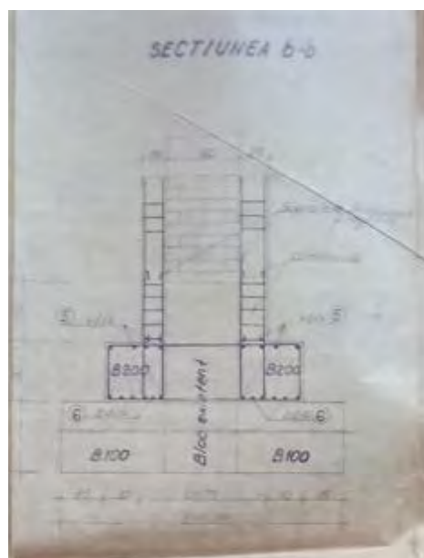
Detaliu Fundatie – Proiect realizate in anul 1977 de ing. Manea T. si ing. Turcanu Ion.
