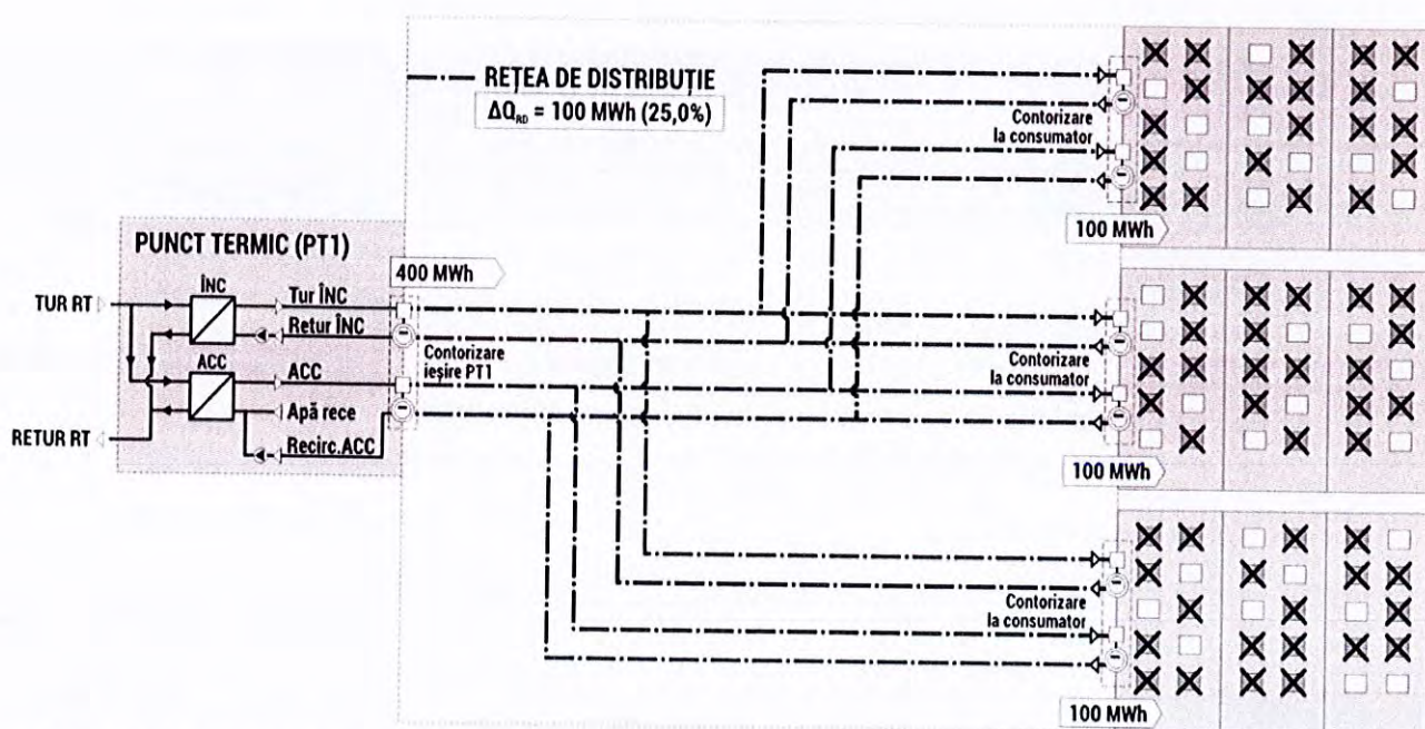
Fig. 8.2. Rețea de distribuție existentă – varianta actuală, la momentul t_2 (2/3 dintre consumatorii inițiali s-au debransat de la rețeaua de distribuție)
