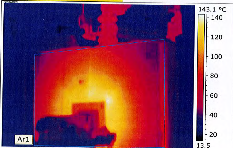
Thermogram: IR_0410.JPG 2/6/2026
