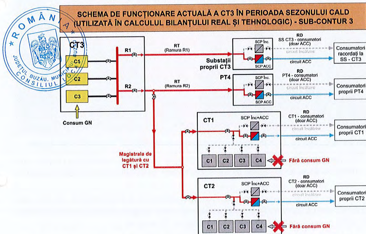
Fig. 2.7. Sub-contur 3: schema de funcționare în sezonul CALD, în perioada de referință a bilanțului (pentru calculul bilanțului real și tehnologic)
