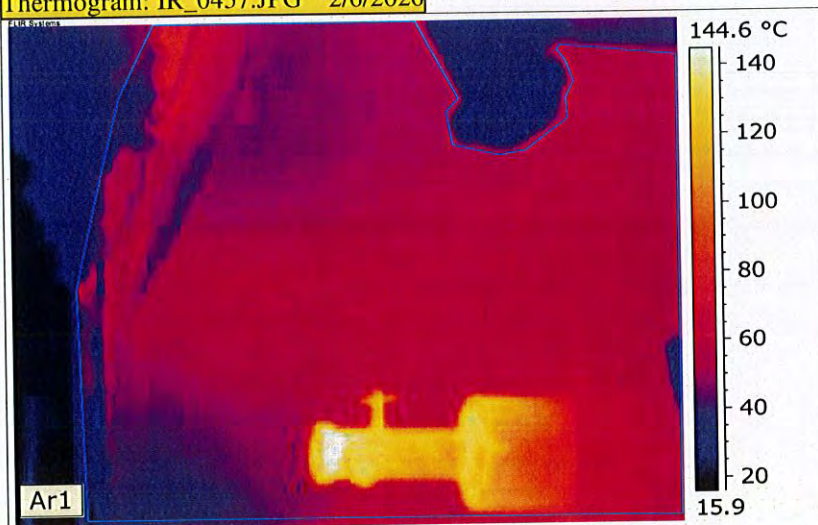
Thermogram: IR_0457.JPG 2/6/2026
