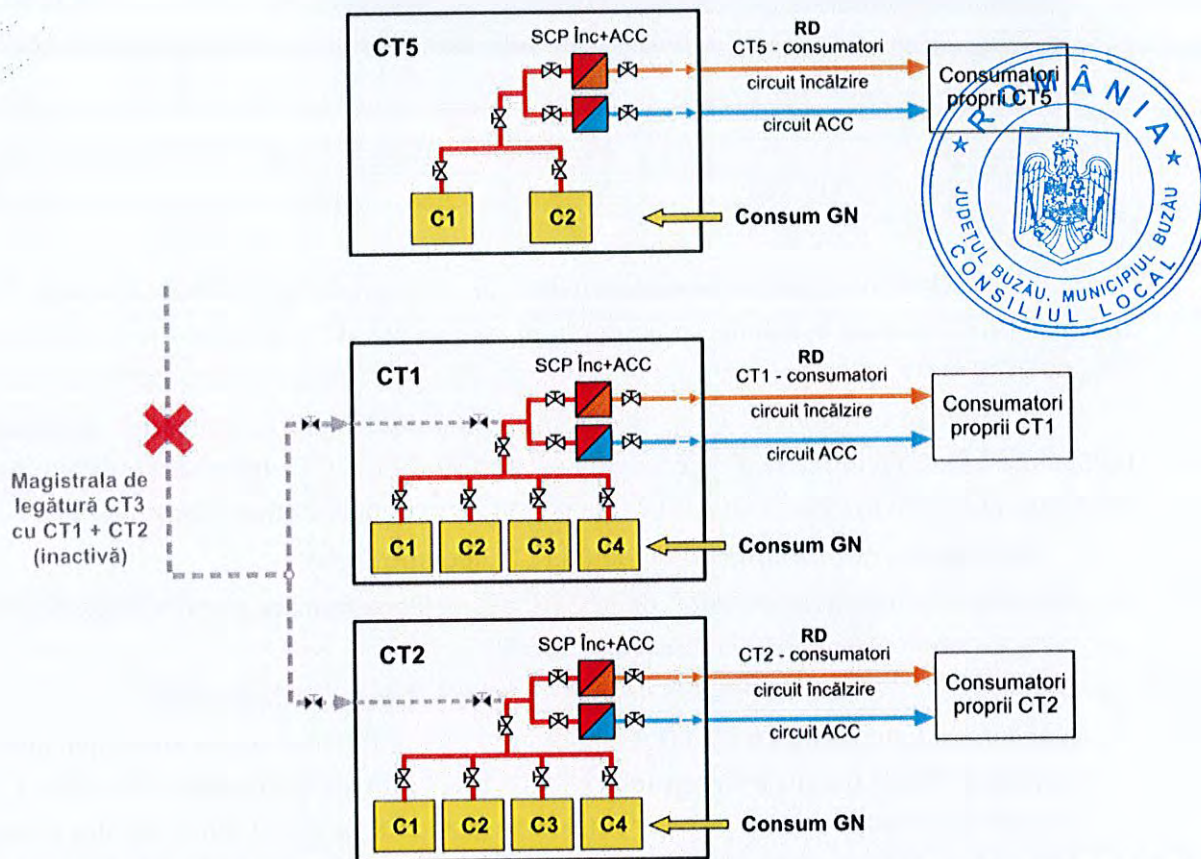
Fig. 2.4. Sub-contur 2: schema de funcționare în sezonul RECE, în perioada de referință a bilanțului (pentru calculul bilanțului real și tehnologic)
