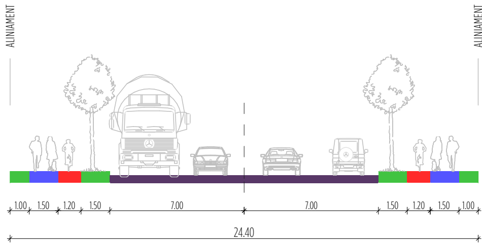
PROFIL TRANSVERSAL SOS. CONSTANTEI - STRADA CATEGORIA II
